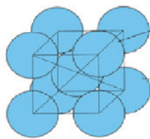
fémes kötés 2
