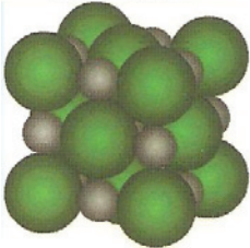
ionos kötés
