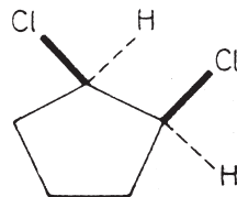
cisz -1,2-diklór-ciklopentán
