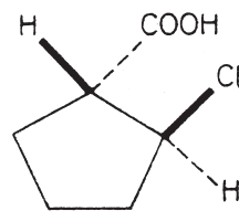
transz -2-klór-1-ciklopentánkarbonsav
